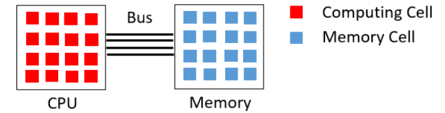
(a) Von Neumann Computing System
